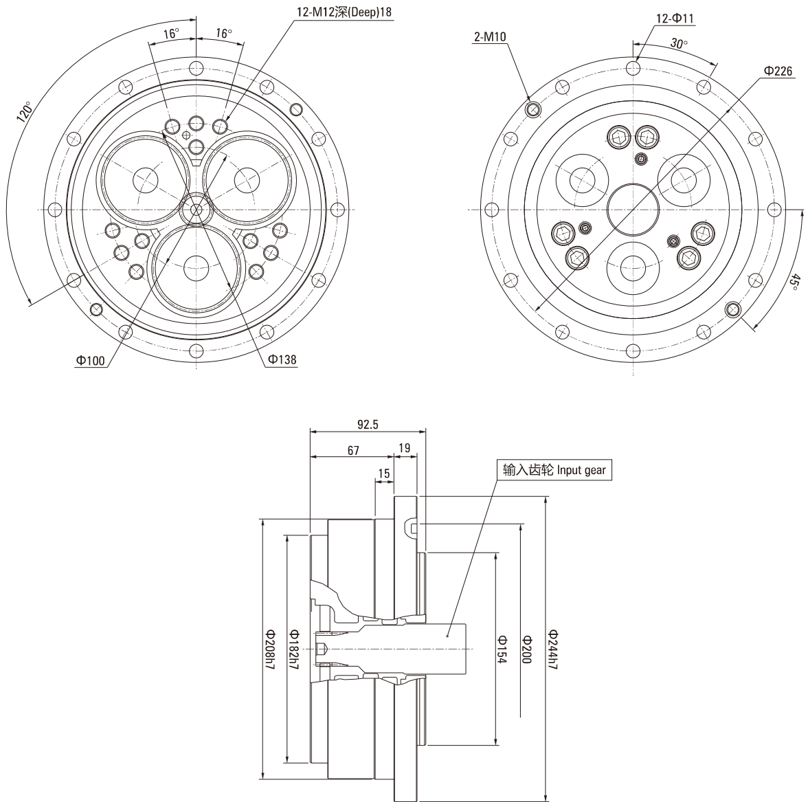
250BX-E 外形图 250BX-E Outline Drawing
