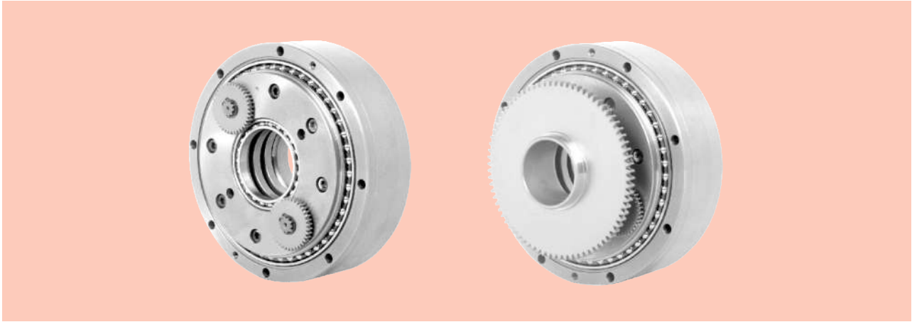
220BX-C 外形图 220BX-C Outline Drawing
