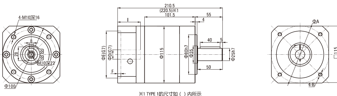
※1 TYPE 1的尺寸如 ( ) 内所示
