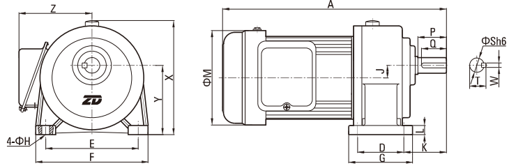
■ 卧式 Horizontal
