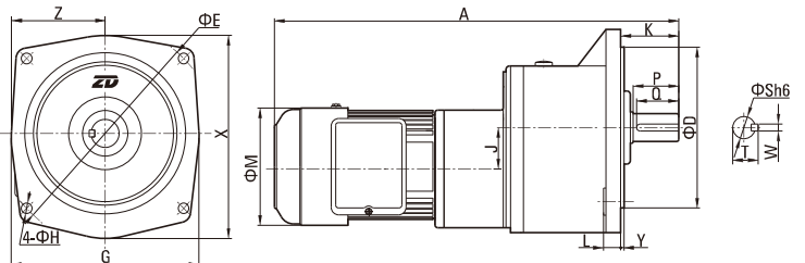
■ 立式 Vertical
